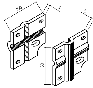
조립구 상세 SCALE: NONE
