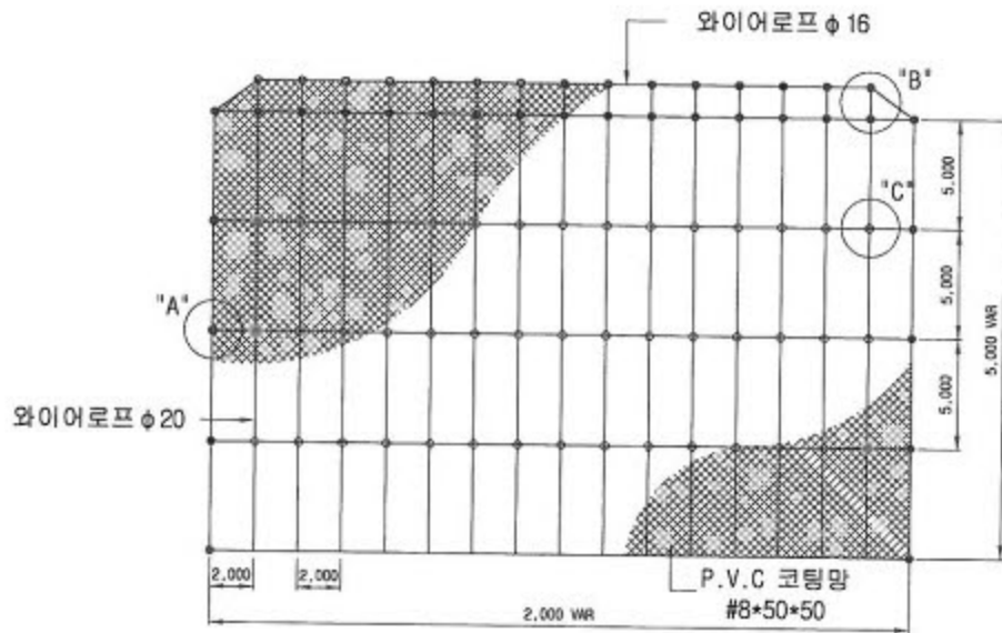
정면 SCALE: NONE
