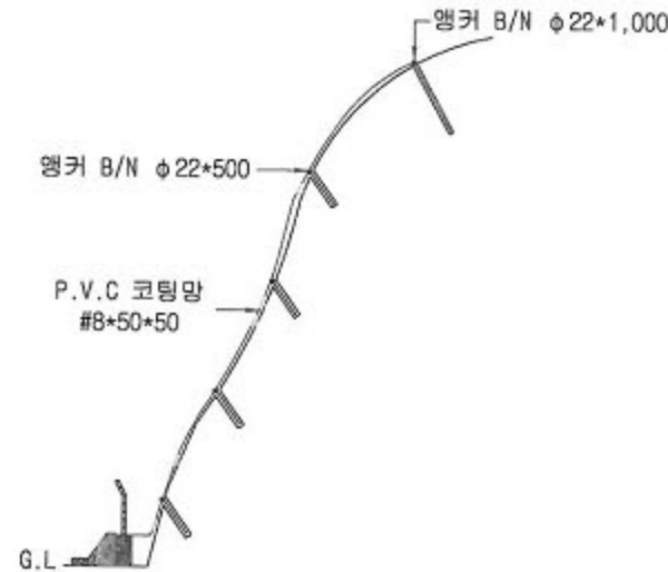
측면 SCALE: NONE
