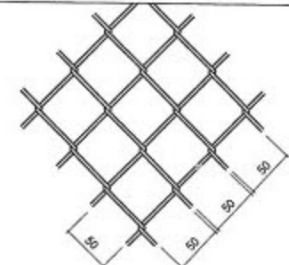
코팅망 상세 SCALE: NONE
