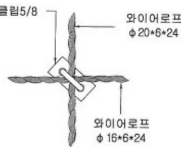
"C" 상세도 SCALE: NONE
