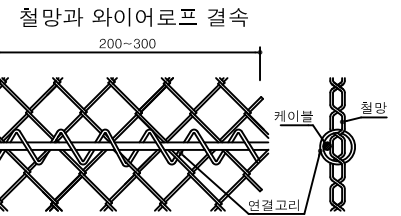
코팅망 상세 SCALE : NONE
