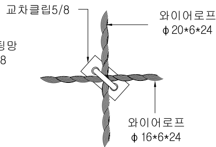
"C" 상세도 SCALE : NONE
