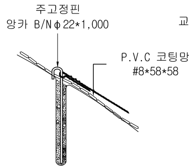
"B" 상세도 SCALE : NONE
