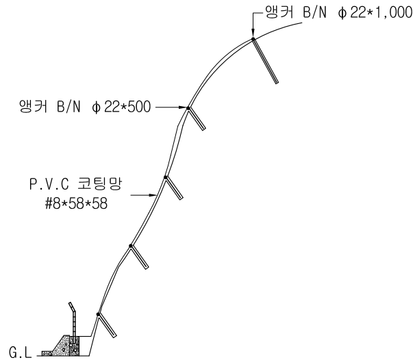
측면 SCALE : NONE
