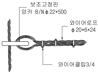
"A" 상세도 SCALE : NONE
