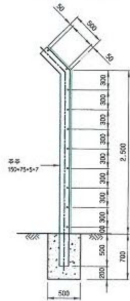
측면도 (중간지주)
