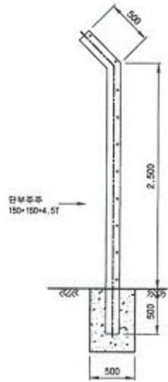
측면도 (단부지주)
