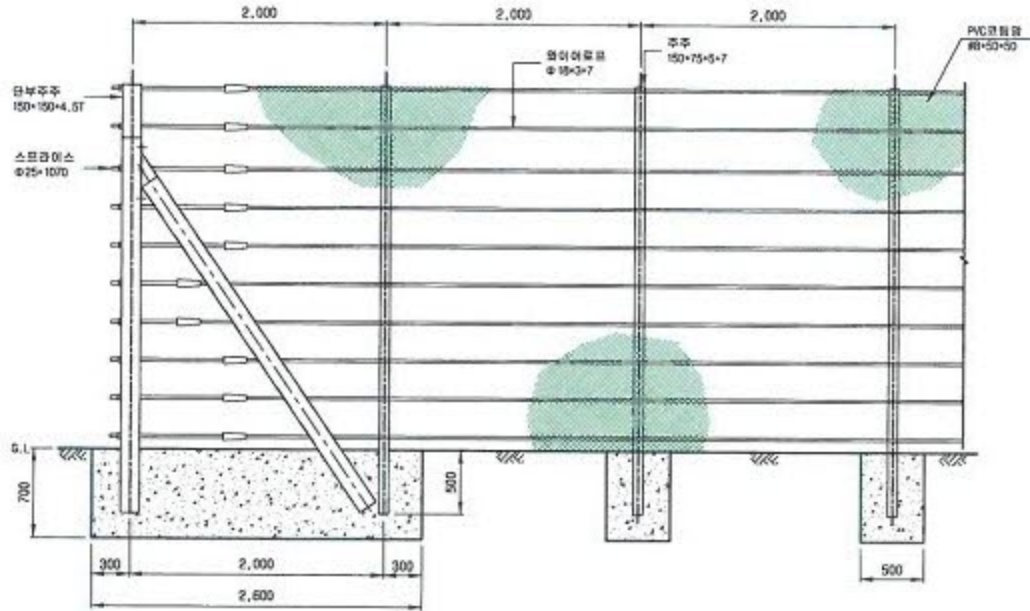
정면도
