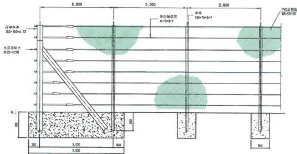
정면도
