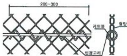
철망과 와이어로프 결속
