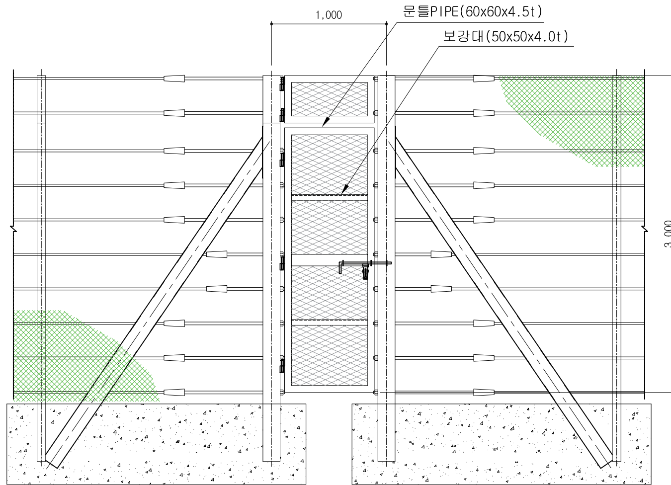
ELEVATION SCALE: NONE
