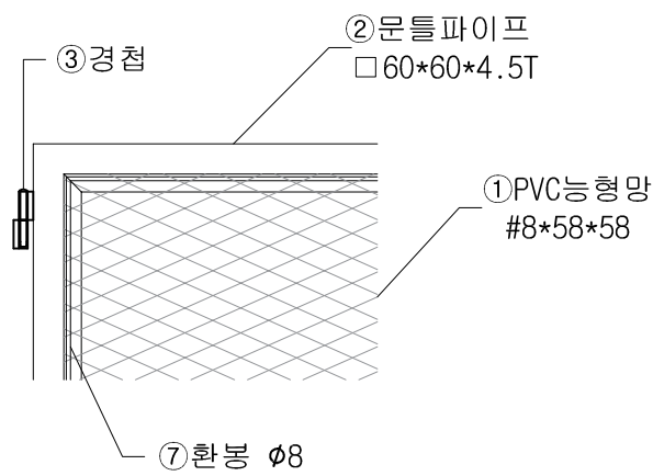
문틀 상세도 SCALE: NONE
