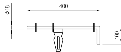
빗장/고리 상세도 SCALE: NONE
